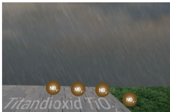
Regenwasser transportiert das Nitrat ( \text{NO}_3^- ) von der Fläche. Das Nitrat dient den Pflanzen als Nährstoff.
